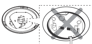
アダプターと本体が斜めにずれている
